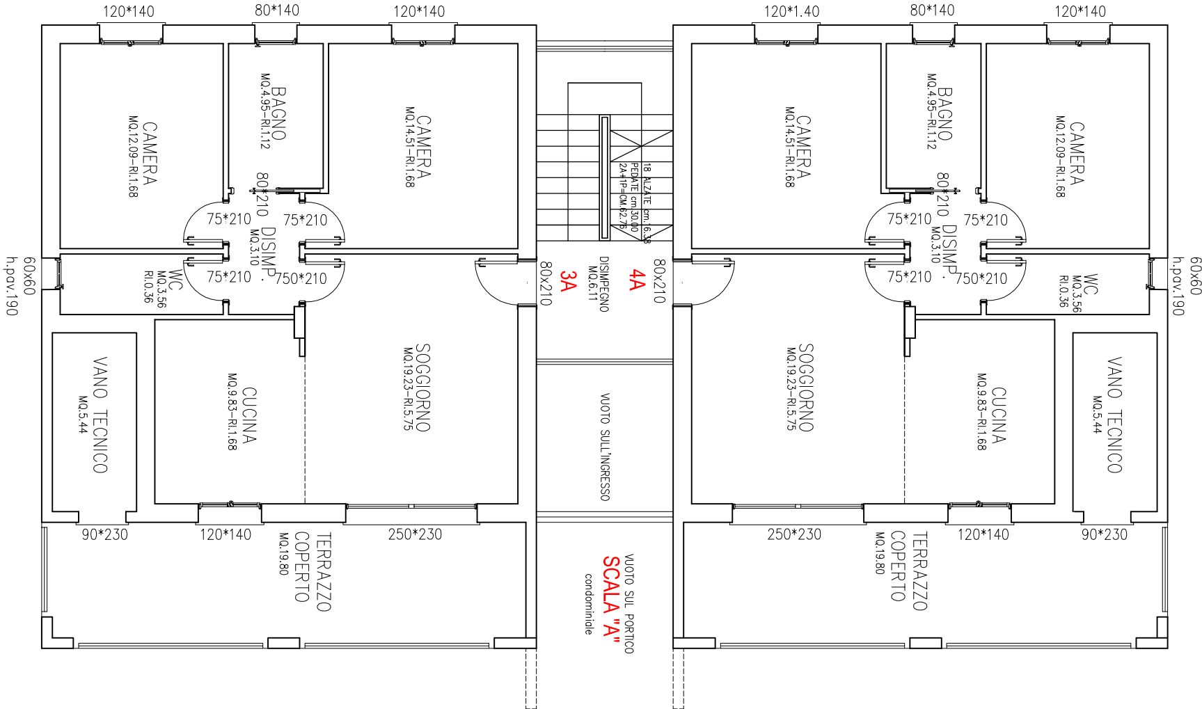
PIANO PRIMO BLOCCO "A"
